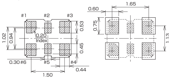
【ランドパターン(参考)】 <TOP View>
