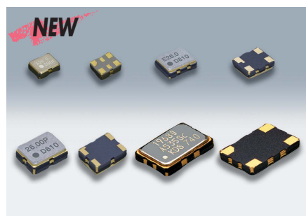
原寸大 DSA211SCA DSA221SCA DSA321SCA DSA535SC DSB211SCA DSB221SCA DSB321SCA DSB535SC
