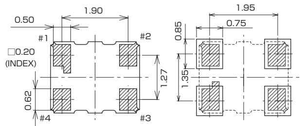
【ランドパターン(参考)】 <TOP View>
